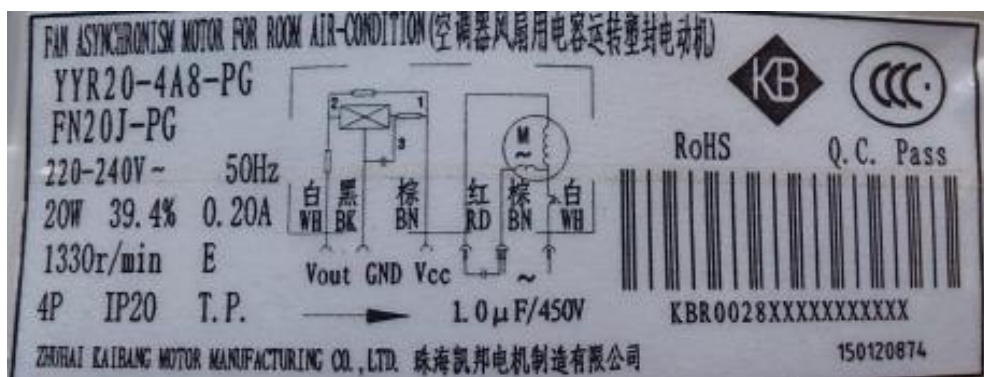
Fan motor marking
