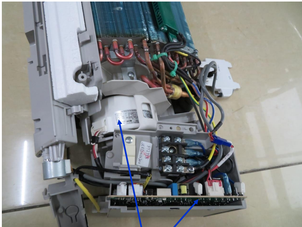
Fan motorMain board
