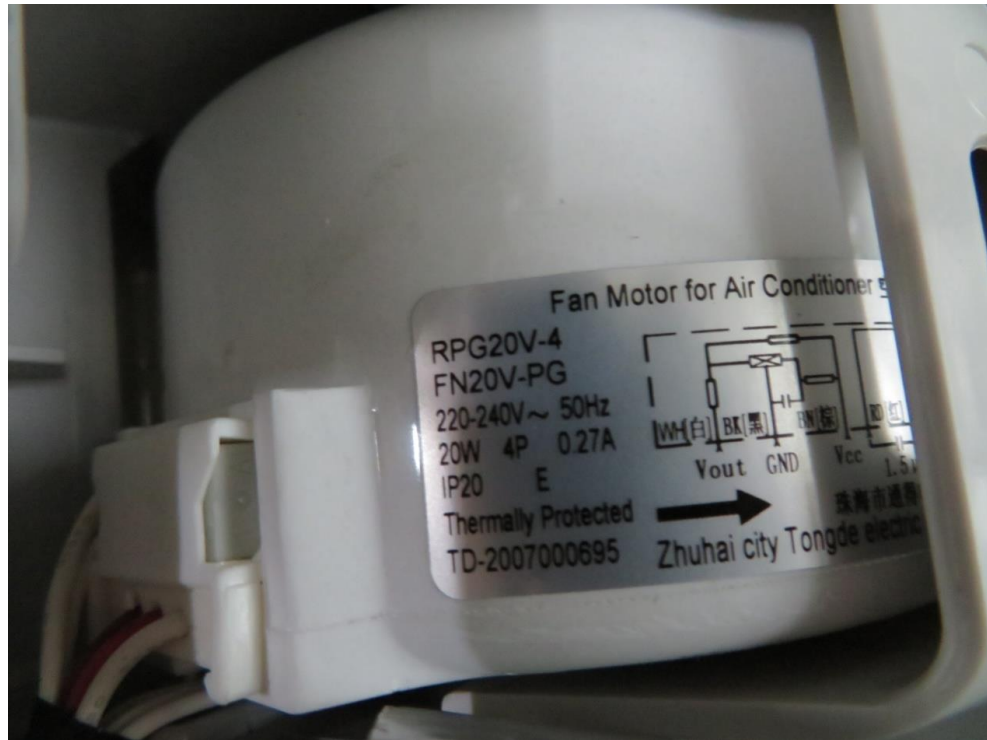
Fan motor
